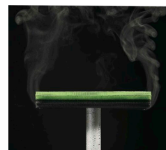
【通気実験】 エアレイヤーベースの下から水蒸気を吹き込んだ状態。波形ループからなる筒型形状によって、湿気が横に抜けやすくなっています。
